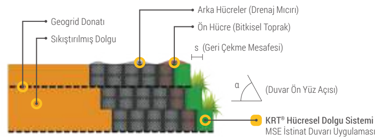
Flexi HDS İstinat Duvarı Enkesit Detayı
